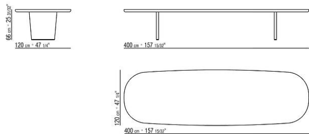
COD. 02F589 TISCH H.66
