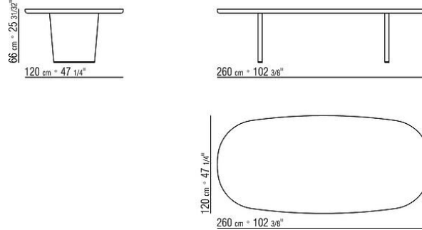
COD. 02F589 TISCH H.66
