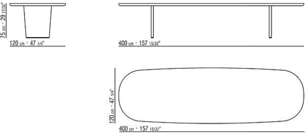
COD. 02F599 TISCH H.75
