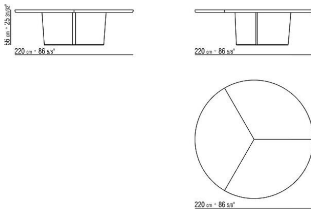
COD. 02F584 TISCH H.66
