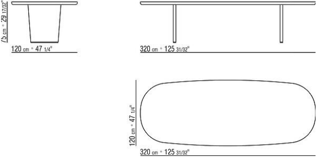
COD. 02F598 TISCH H.75
