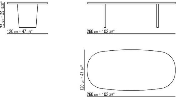
COD. 02F599 TISCH H.75
