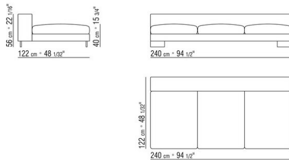
COD. 011P12 ELEMENT / DACRON
