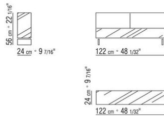
COD. 011P92 KISSEN
