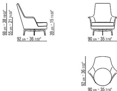
COD. 015M41 SOFT-SESSEL METALLGESTELL DREHBAR
