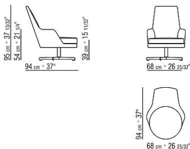
COD. 015M11 GA.11-SESSEL METALLGESTELL DREHBAR
