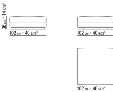
COD. 014V53 HOCKER ZWISCHENELEMENT
