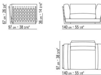
COD. 014L61 SOFA RUECK/GEPOLST ARM/KERNLEDER
