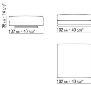
COD. 014V55 HOCKER ZWISCHENELEMENT
