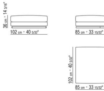
COD. 014V62 SOFA RUECK/GEPOLST ARM/KERNLEDER
