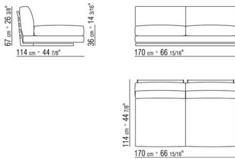
COD. 014V15 ECKELEMENT / ENDELEMENT L / KERNLEDER
