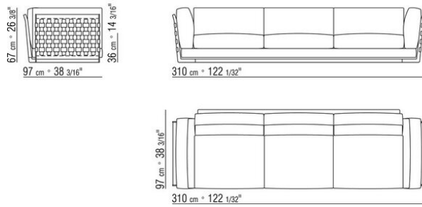
COD. 014L72 ELEMENT / GEPOLSTERT
