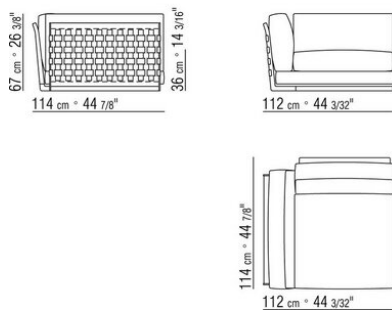
COD. 014V79 ECKENELEMENT L RUECK/GEPOL ARM/KERN
