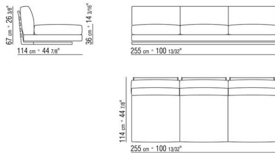
COD. 014V17 ECKELEMENT / ENDELEMENT L / KERNLEDER
