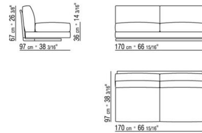
COD. 014L72 ELEMENT / GEPOLSTERT
