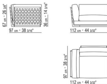
COD. 014L15 ECHELEMENT / ENDELEMENT L / KERNLEDER
