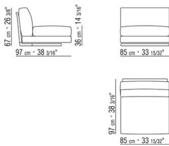
COD. 014L73 ELEMENT / GEPOLSTERT
