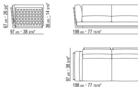
COD. 014L17 ECHELEMENT / ENDELEMENT L / KERNLEDER
