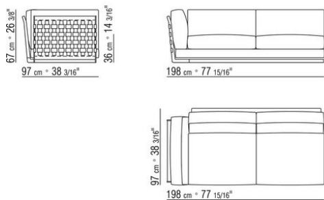
COD. 014L77 ECKENELEMENT L RUECK/GEPOL ARM/KERN
