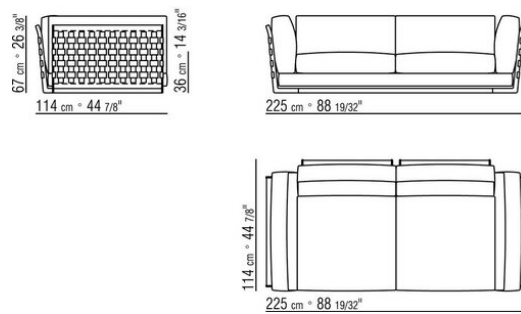
COD. 014V02 SOFA / KERNLEDER
