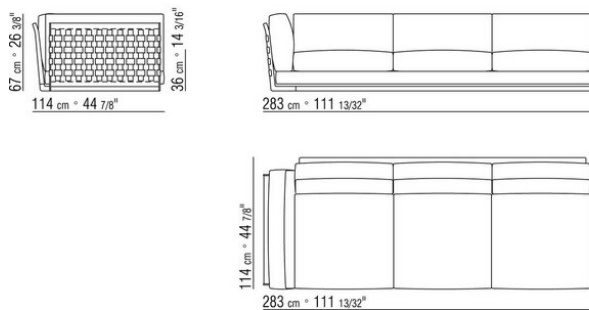
COD. 014V79 ECKENELEMENT L RUECK/GEPOL ARM/KERN
