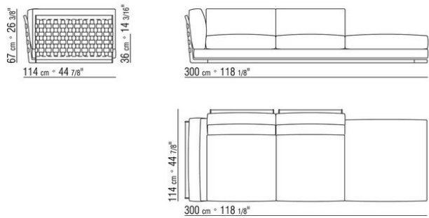
COD. 014V95 LANGE ECKE L / RUECK/KERNLEDER ARM/GEPOLST
