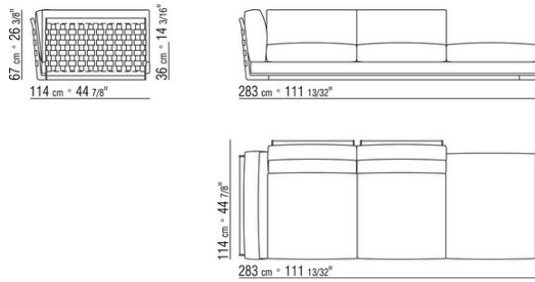
COD. 014V29 LANGE ECKE L / RUECK/KERNLEDER ARM/GEPOLST
