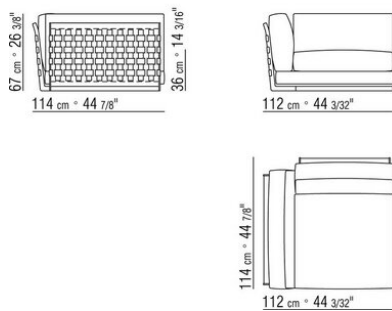
COD. 014V19 ECKELEMENT / ENDELEMENT L / KERNLEDER
