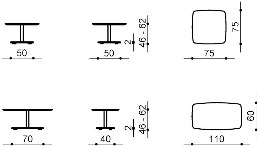
Couchtisch mit bombierter quadratischer oder rechteckiger Platte
