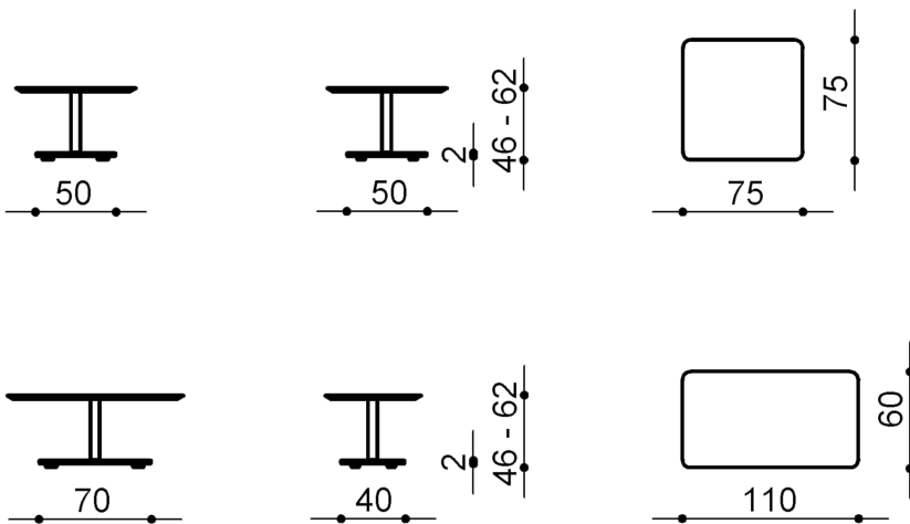
Couchtisch mit quadratischer oder rechteckiger Platte mit Rundercken
